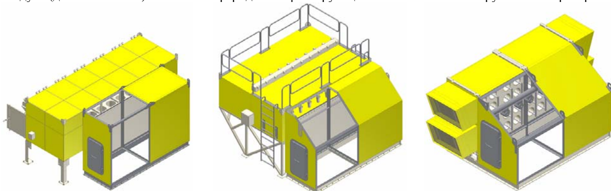
Рис. №3 КВОУ на расход воздуха 80000 м 3 /ч с фильтрующими элементами Camfil Farr GS.
